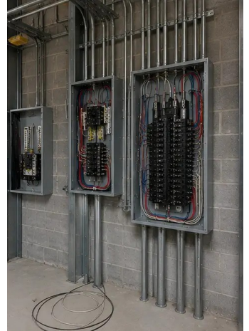
Ảnh số11. Lắp đặt hệ thống điện đang tiến hành
