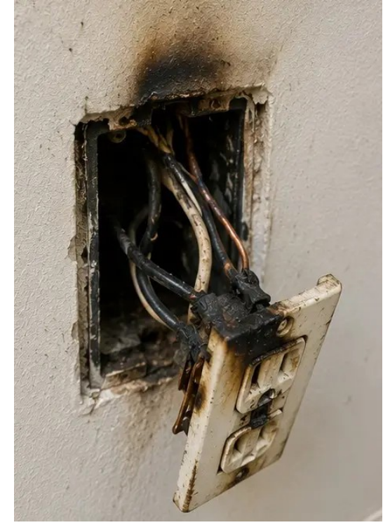
Görüntü No12 Denetim sırasında kaydedilen elektrik sistemi hasarı
