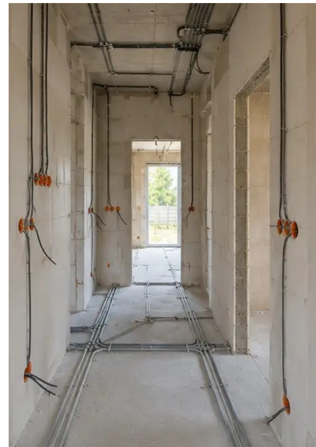
Слика бр.9 Инсталација електричних система у току
