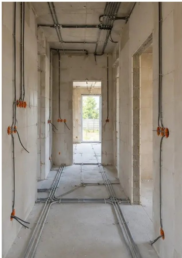
Слика бр.9 Инсталација електричних система у току
