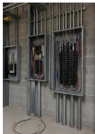
Слика бр.11. Инсталација електричних система у току
