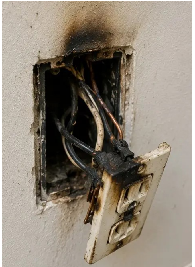
Foto št.12 Poškodba električnega sistema zabeležena med pregledom
