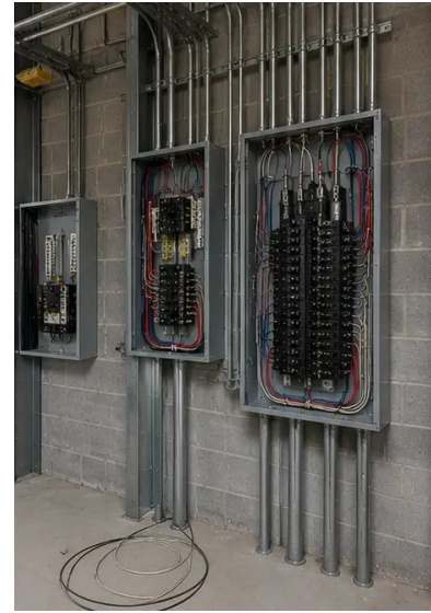
Fotografia č. 11. Inštalácia elektrických systémov prebieha
