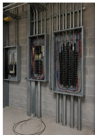
Фото №11. Монтаж электрических систем в процессе
