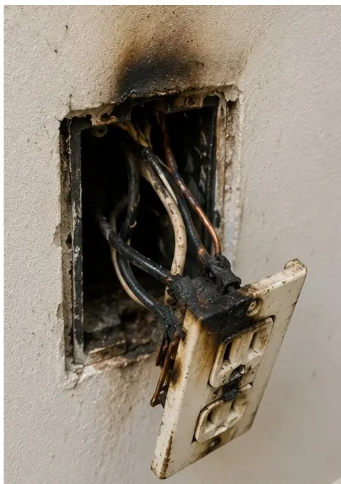
Foto nº12 Dano no sistema elétrico registado durante a inspeção
