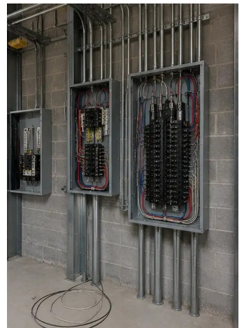
Foto №11. Installatie van elektrische systemen in uitvoering
