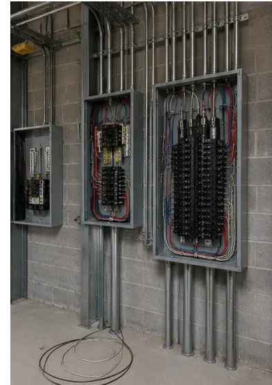
Foto №11. Installatie van elektrische systemen in uitvoering
