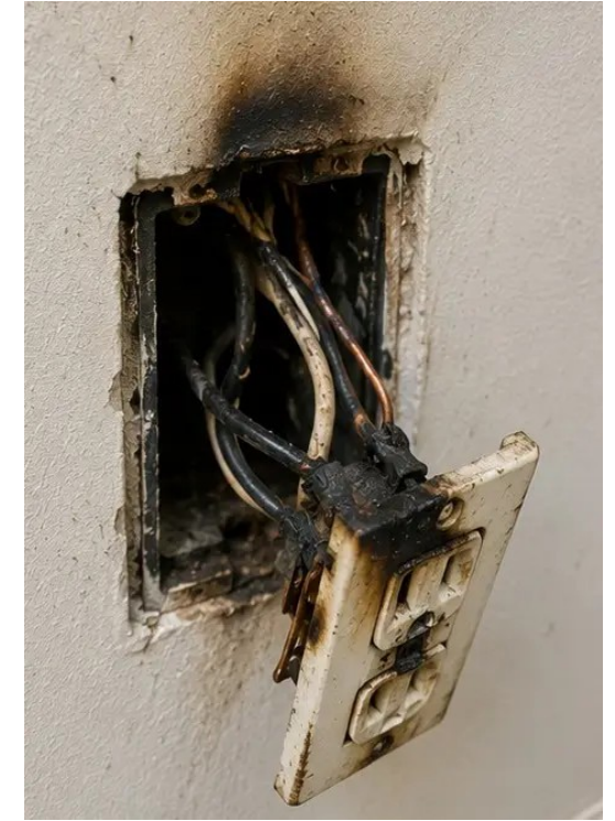
Foto №12 Kerusakan sistem kelistrikan tercatat selama inspeksi
