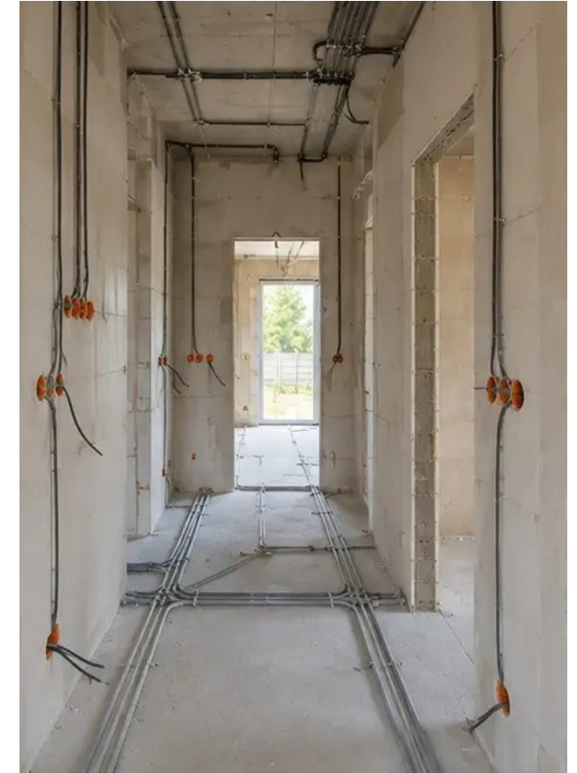
Fotografija br.9 Instalacija električnih sustava u tijeku
