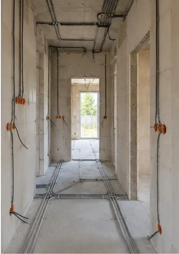
Φωτογραφία Νο9 Εγκατάσταση ηλεκτρικών συστημάτων σε εξέλιξη
