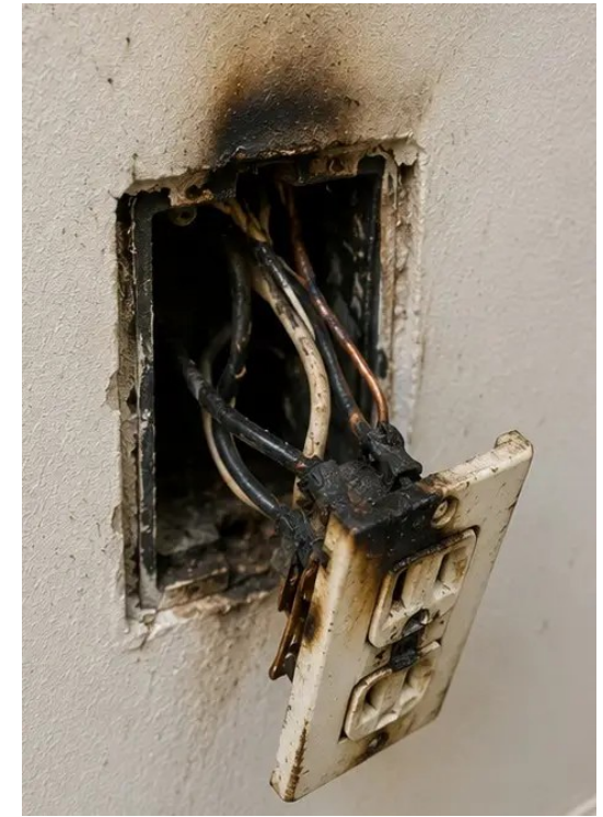
Fotografie č. 12 Poškození elektrického systému zaznamenáno během prohlídky
