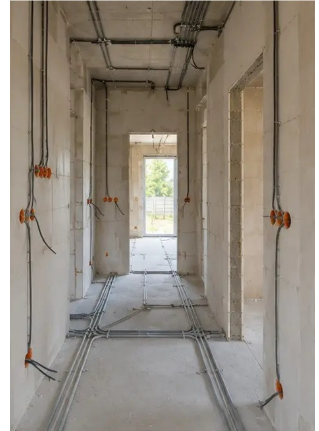
Fotografie č. 9 Probíhá instalace elektrických systémů
