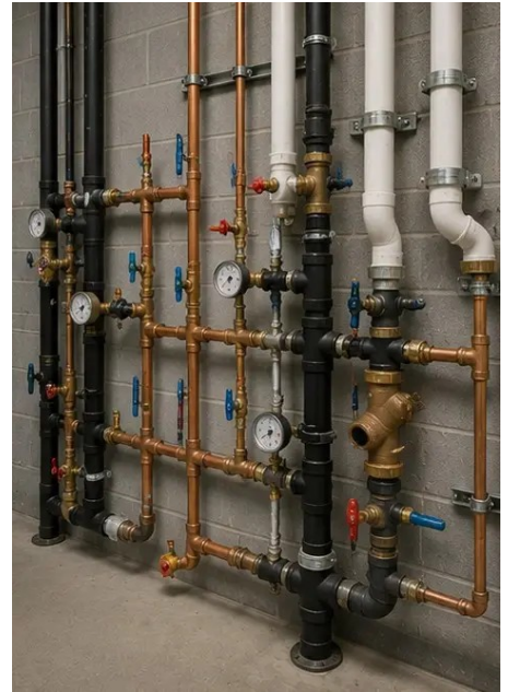
Photo #10. Kontrola instalatérského systému dokončena
