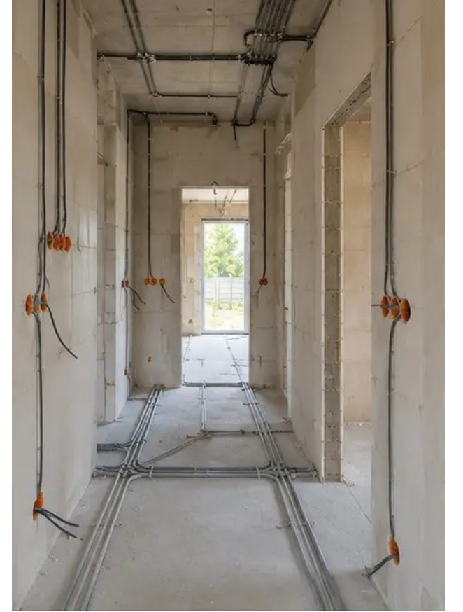
ফটো নং9 ইলেকট্রিক্যাল সিস্টেম ইনস্টলেশন চলছে
