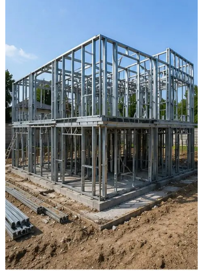
ফটো নং6 স্ট্রাকচারাল ফ্রেম অ্যাসেম্বলি চলছে
