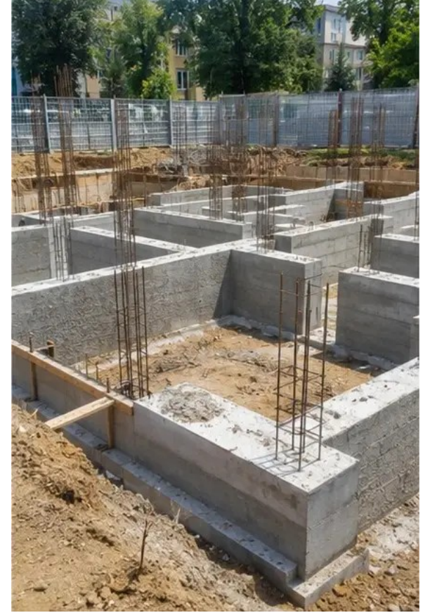
ফটো নং3 ফাউন্ডেশন নির্মাণ চলছে
