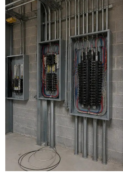
ফটো নং১১. ইলেকট্রিক্যাল সিস্টেম ইনস্টলেশন চলছে
