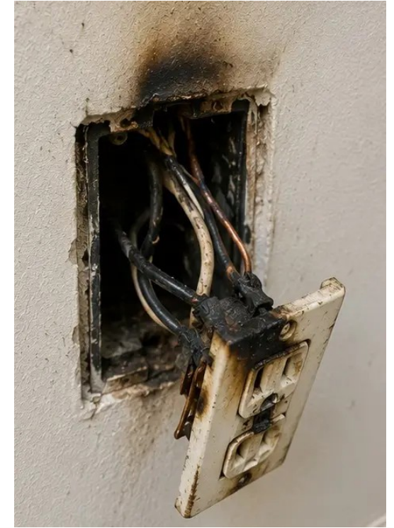
Снимка №12 Щети по електрическата система, записани при инспекцията
