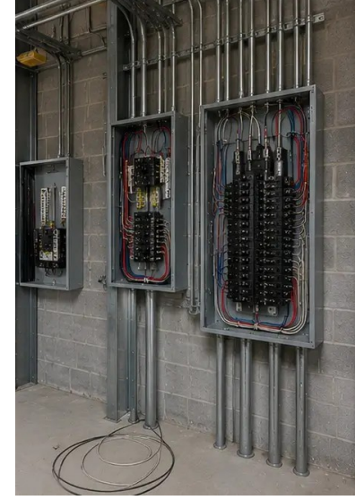
صورة رقم 11. تركيب الأنظمة الكهربائية قيد التنفيذ
