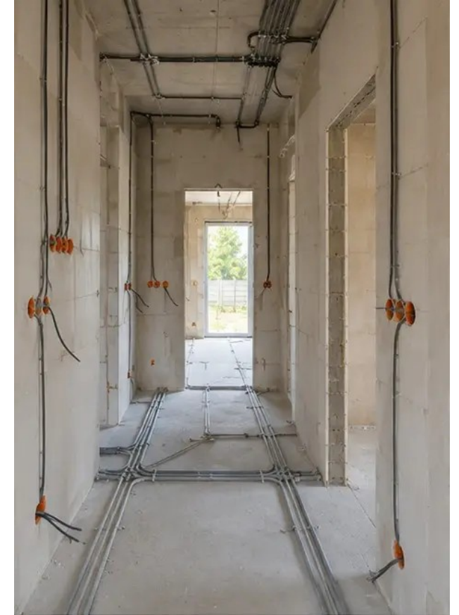
صورة رقم 9 تركيب الأنظمة الكهربائية قيد التنفيذ
